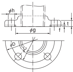
固定フランジ
