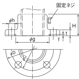
摺動フランジ
