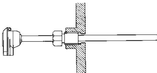
固定ニップル取付
