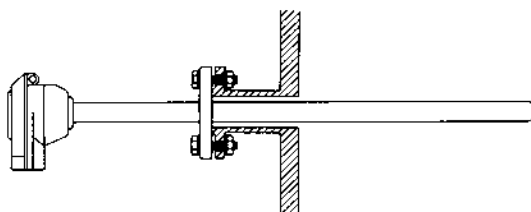
固定フランジ取付
