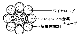
●断面図
