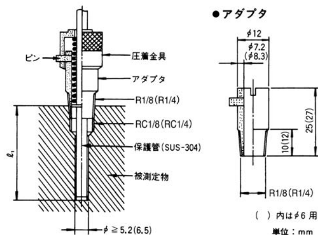
スプリング圧着取付
